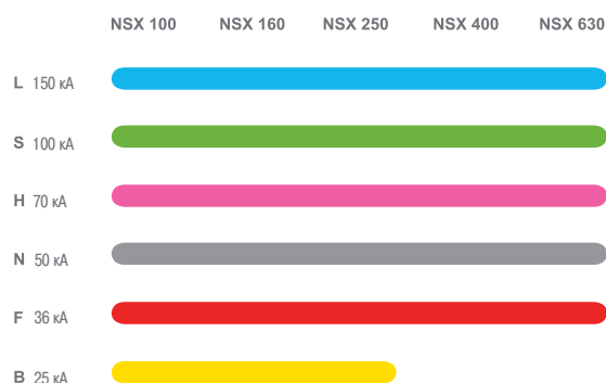
Уровни отключающей способности при 415 В
