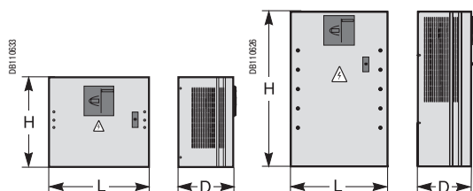
Шкаф с автоматическим выключателем, типоразмер С1
