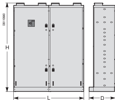
Шкаф без автоматического выключателя, типоразмер A4
