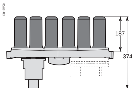
Размеры Varpact CLASSIC и CLASSIC B
