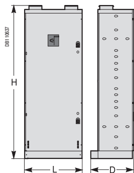
Шкаф без автоматического выключателя, типоразмер A3
