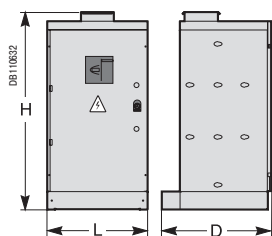
Шкафы без автоматического выключателя, типоразмеры A1 и A2
