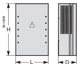
Шкаф без автоматического выключателя, типоразмер C2
