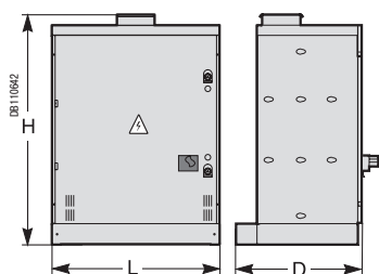
Шкаф с автоматическим выключателем, типоразмер A2
