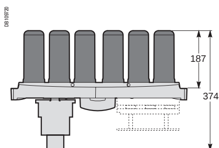
Размеры Varpact COMFORT и COMFORT B
