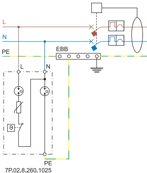
ТТ-ОДНОФАЗНАЯ СИСТЕМА - УСТАНОВКА SPD ДО УЗО
