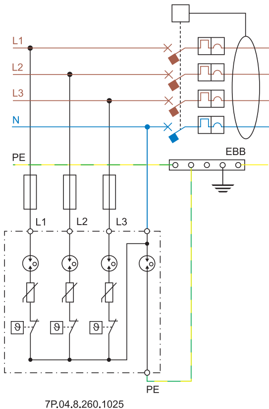
ТТ-ТРЕХФАЗНАЯ СИСТЕМА - УСТАНОВКА SPD ДО УЗО
