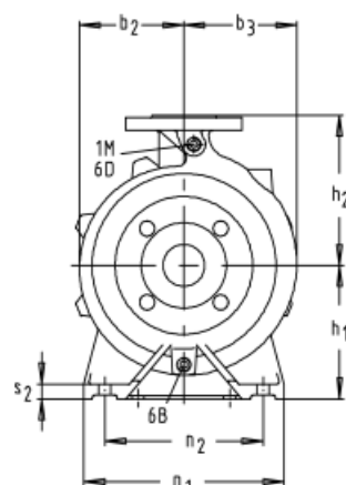
Etanorm C
