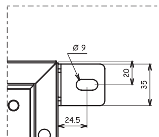
Уголок для монтажа к стене
