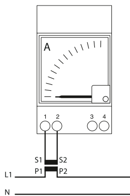
Включение через трансформатор тока
