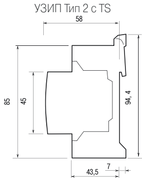
2 полюса (1P+N)
