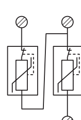
OVR 2 15 75
