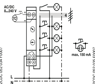
Е 232Е-8/230 Multi 10 4 - проводная схема
