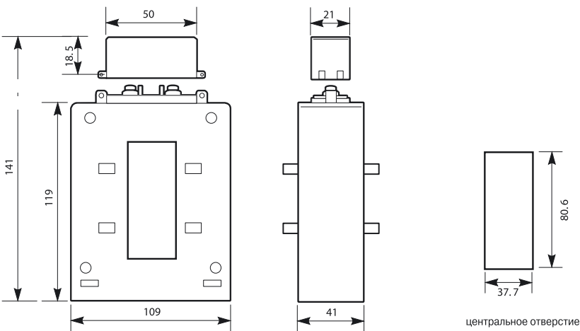
CT8-V
