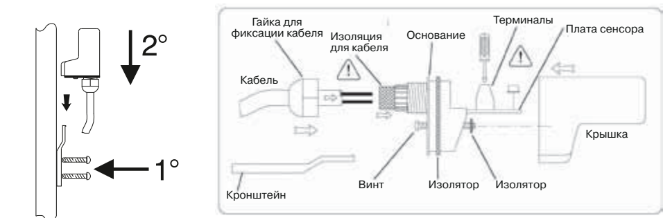
Схема датчика
