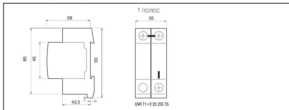
УЗИП Тип 1 и Тип 1+2 ( I_{fi} = 7 \text{ кА} )
