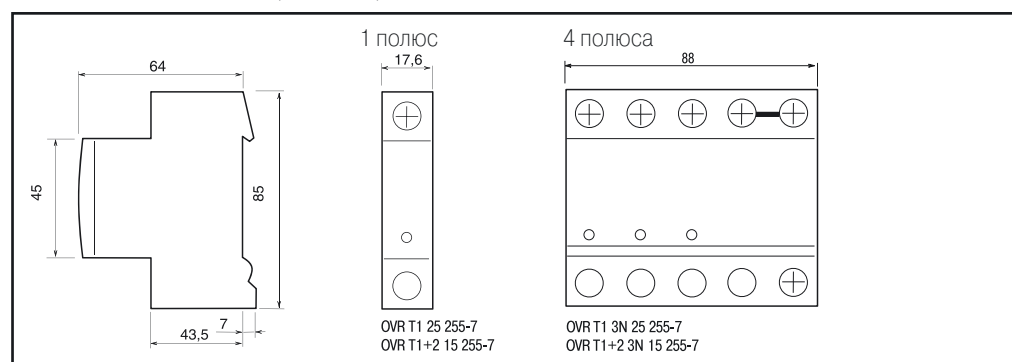
УЗИП Тип 1 и Тип 1+2 ( I_{fi} = 7 \text{ кА} )
