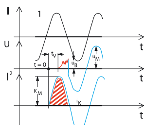
Автоматический выключатель без ограничения тока
