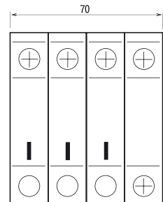
3 полюса (3P+N)
