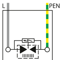
OVR T1 25 440-50
