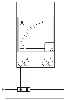
Включение через шунт
