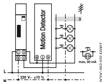
E 232E-8/230 Multi 10 3 - проводная схема
