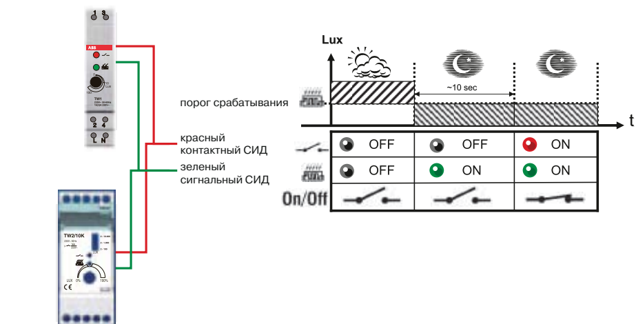
TW1 и TW2/10K принцип работы
