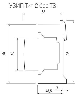
1 полюс
