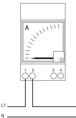
Прямое включение
