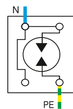
OVR T1 100 N
