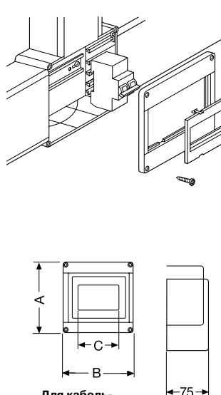
Кожух для установки модульных устройств размером 17,5x45 мм
