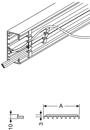
Кабельный фиксирующий элемент
