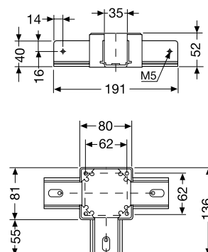
Плоский крестообразный отвод
