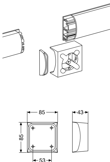
Коробка для выключателей/розеток с расстоянием между центрами отверстий 60/67 мм
