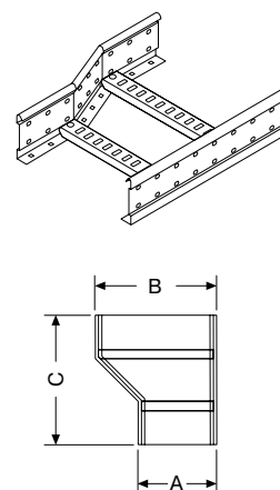
Левостороннее соединение с сужением
