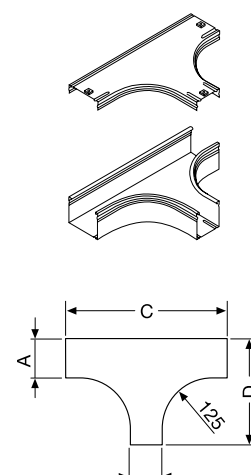
Плоский Т-образный отвод с сужением
