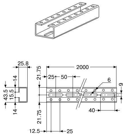
Подвесная рейка С-образного профиля
