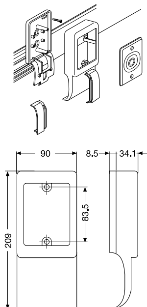
Вертикальная коробка для выключателей/ розеток
