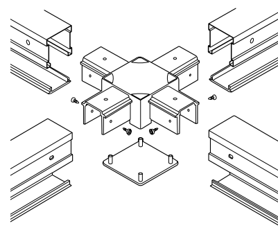
Плоский крестообразный отвод
