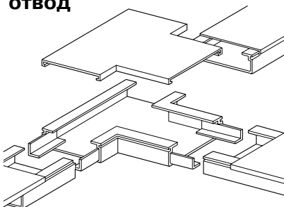
Плоский Т-образный отвод
