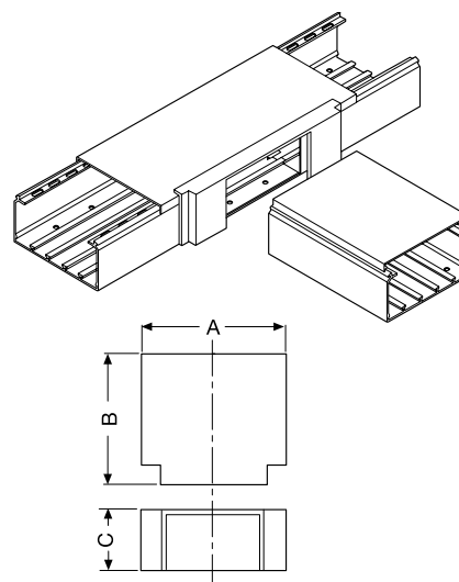
Плоский Т-образный отвод
