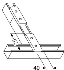
Плоские перфорированные фиксирующие пластины
