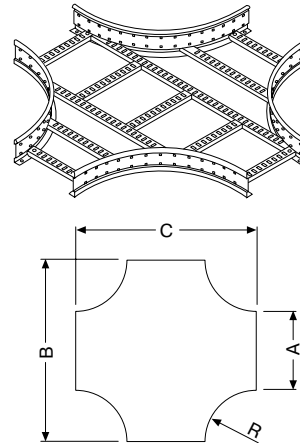
Плоский крестообразный отвод
