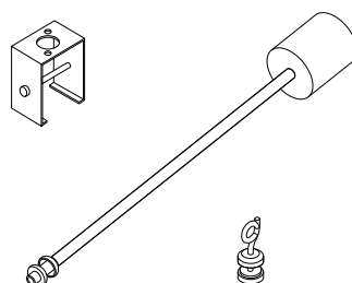
Опора, гак и стержень с резьбой для подвеса кабель-канала
