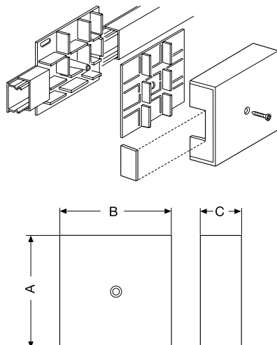
Распаячная коробка для выполнения плоских отводов
