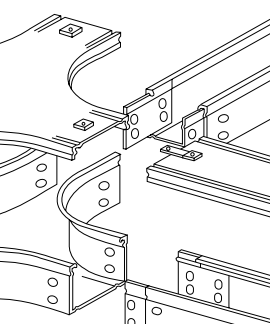
Плоский крестообразный отвод
