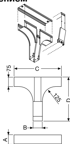
Вертикальный Т-образный отвод с сужением
