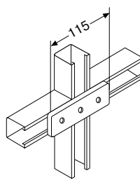
Плоские перфорированные фиксирующие пластины
