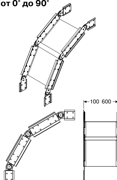
Восходящие и нисходящие навесные сегменты, с регулируемым углом от 0° до 90°
