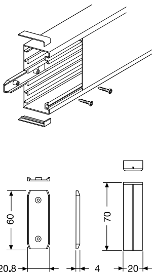
Плоское соединительное звено для кабель-каналов
