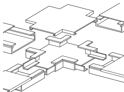
Плоский крестообразный отвод
