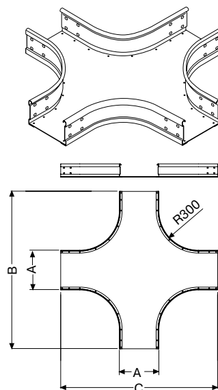
Плоский крестообразный отвод
