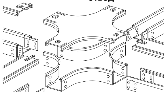
Плоский крестообразный отвод
