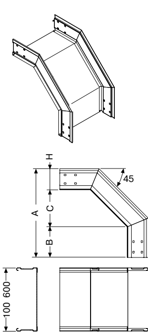
Нисходящий угловой сегмент 90°
