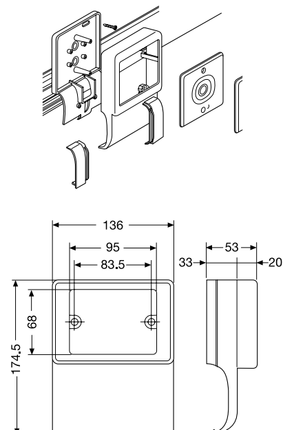
Горизонтальная коробка для выключателей/ розеток
