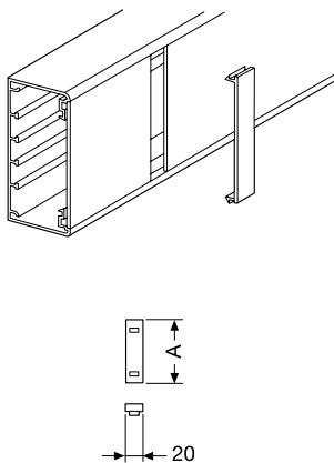
Соединительная скоба для крышек
