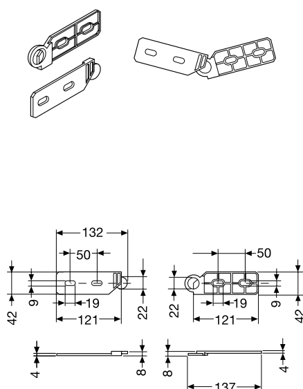
Регулируемое соединительное звено
