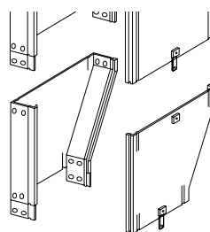
Лево- и правосторонние сужающие соединительные элементы
