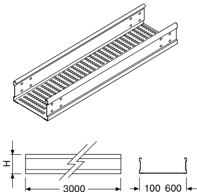
Кабельный лоток с перфорированным основанием
