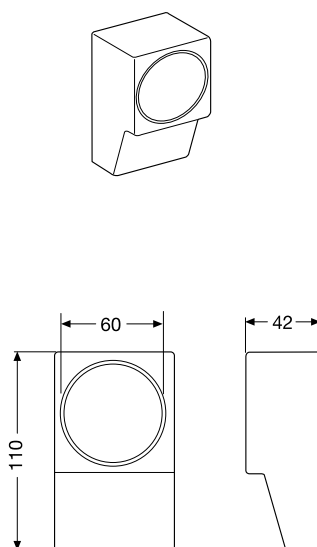
Напольная коробка для выключателей/ розеток Ø 60 мм
