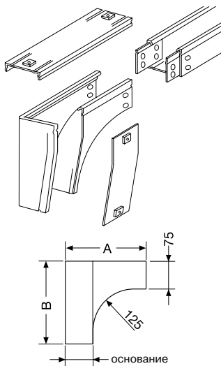
Правый нисходящий угловой сегмент 90°
