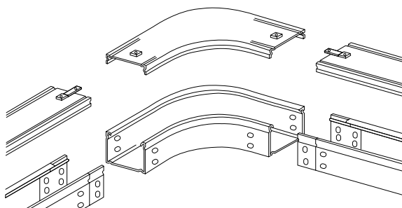
Плоский угловой сегмент 90°
