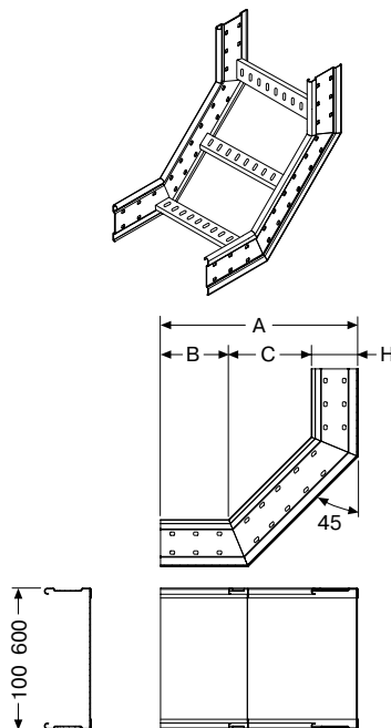
Восходящий угловой сегмент 90°
