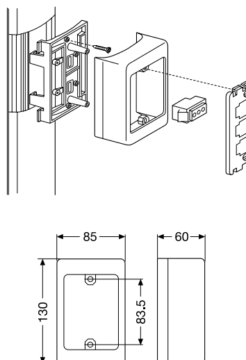
Коробка для выключателей/розеток с расстоянием между центрами отверстий 83,5 мм
