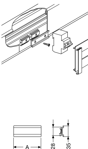
Установочный комплект для модульных устройств
