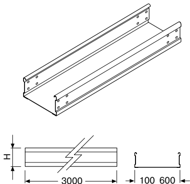
Кабельный лоток с глухим основанием
