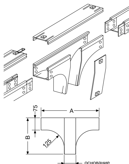
Вертикальный Т-образный отвод с выравнивающим сдвигом
