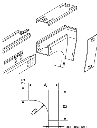
Левый нисходящий угловой сегмент 90°
