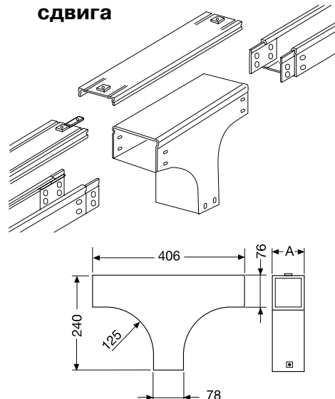
Вертикальный Т-образный отвод без выравнивающего сдвига
