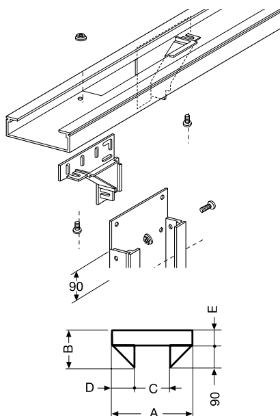
Элемент для подсоединения отвода
