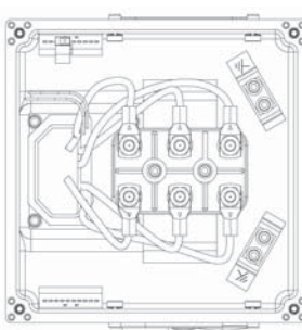
Соединительная коробка для типоразмеров двигателя 200–280
