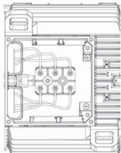
Соединительная коробка для типоразмеров двигателя 160–180
