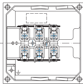
Соединительная коробка для типоразмеров двигателя 90–100
