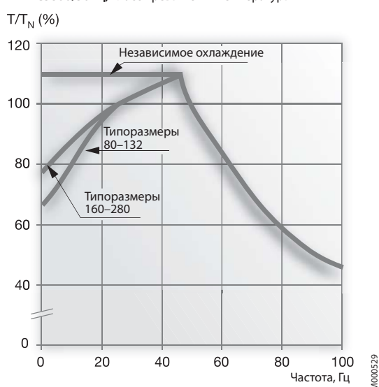
Рис. 4. Нагрузочные кривые с преобразователями ACS550 (электродвигатели промышленного назначения с алюминиевой станиной)
