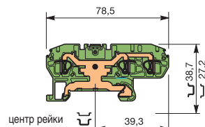
D 4/6.P.3L
