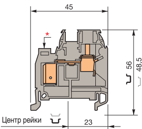
D 6/8.ADO3
