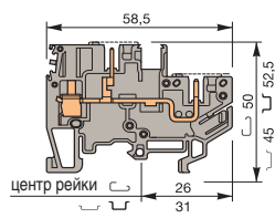
MA 2,5/5.2CPE
