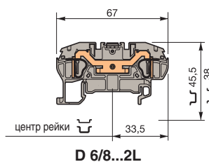
D 6/8...2L
