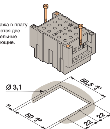
Монтаж в плату Монтаж в стойку
