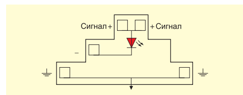
D 2,5/6.DPL1
