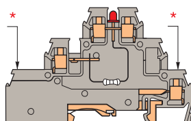
D 2,5/6.DPL1
