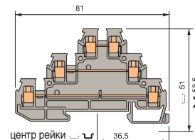
D 2,5/6.DA
