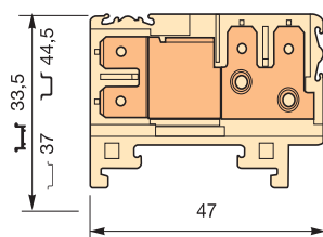
HD 6/8.2G.2G.2
