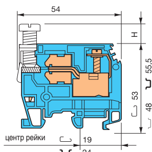
M 16/12.NT1
