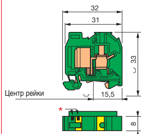
DR 4/8.ADO
