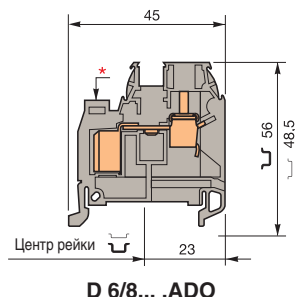
D 6/8... ADO
