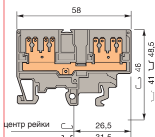
M 2,5/6.4G.1
