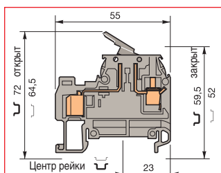
D 2,5/5.SN.ADO
