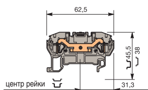
D 4/6.2L
