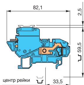
D 6/8.NT.L
