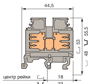
M 2,5/6.2G.2G
