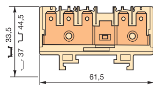
HD 6/9.5G
