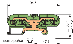
D 4/6.P.4L
