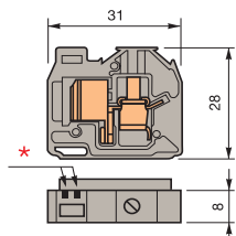
DB 4/8.ADO
