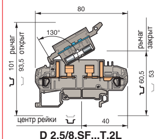
D 2,5/8.SF...T.2L
