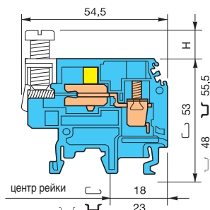
M10/10.NT
