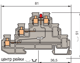
D 2,5/6.DL1
