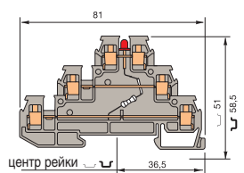
D 2,5/6.DAL1
