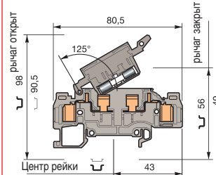
D 2,5/8.SFT.ADO2
