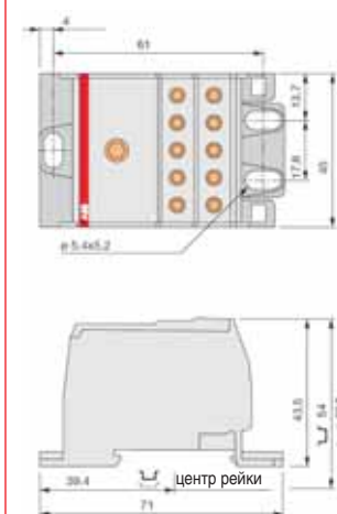
BRU 175
