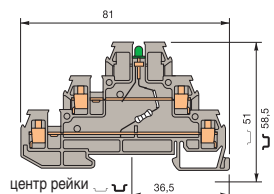
D 2,5/6.DAL2
