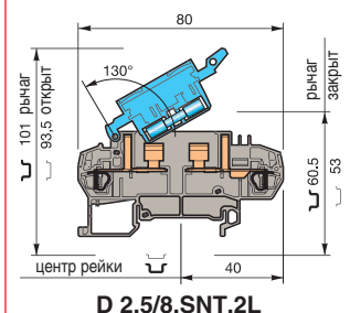
D 2,5/8.SNT.2L
