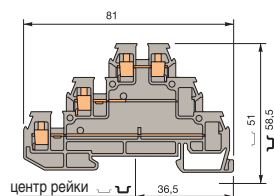
D 2,5/6.D
