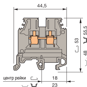
М 4/6
