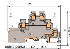
D 2,5/6.DPA1
