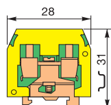
DR 4/6.P
