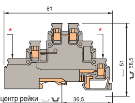
D 2,5/6.DP1
