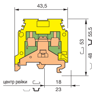
М 4/6.P
