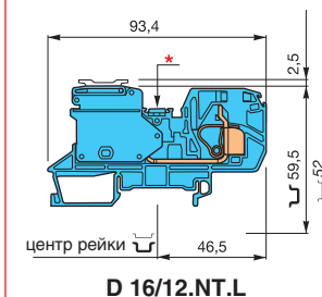
D 16/12.NT.L
