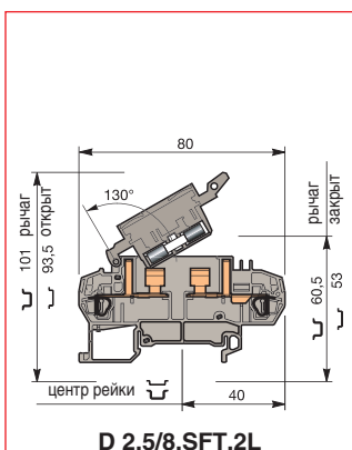
D 2,5/8.SFT.2L
