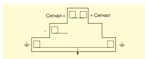
D 2,5/6.DP1
