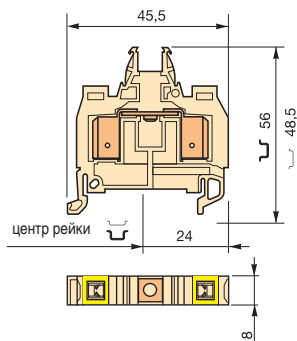
D 4/8.ADO.NF
