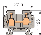
DR 1,5/5
