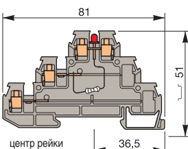
D 2,5/6.DL
