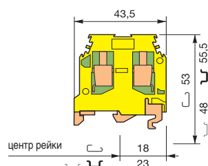
М 6/8.P
