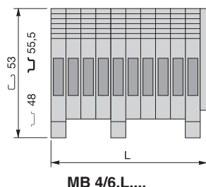
MB 4/6.L....
