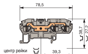
D 4/6.3L
