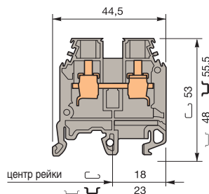
М 6/8
