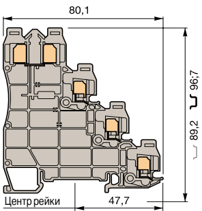
D 1/5.C4.ADO
