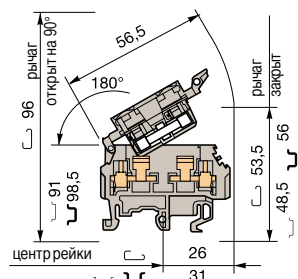
М 4/8.SF
