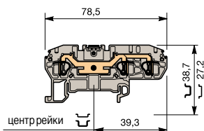
D 4/6.3L
