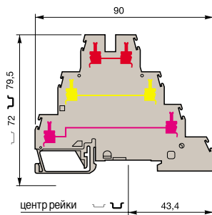
М 4/6.T3
