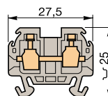
DR 1,5/5
