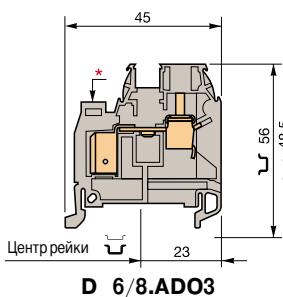
D 6/8.ADO3
