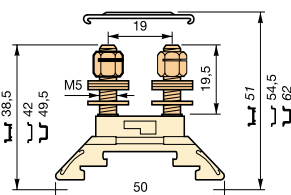
HD10/12.FF5
