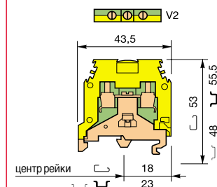
MA 2,5/5.P
