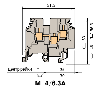
М 4/6.3А
