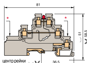
D 2,5/6.DPAL1
