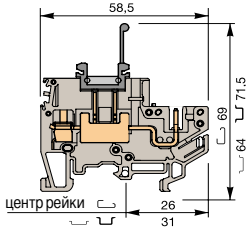
MA 2,5/5-SFA-CPE
