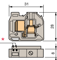
DB 4/8.ADO
