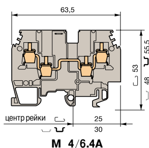
М 4/6.4А
