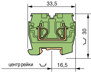
DR 2,5/10.P.4L
