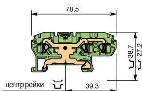
D 4/6.P.3L
