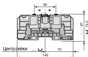
D 70/32.FF
