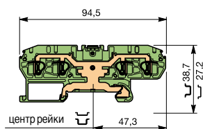
D 4/6.P.4L
