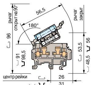
М 4/8.SFL
