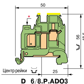
D 6/8.P.ADO3
