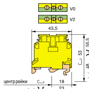
М 10/10.P
