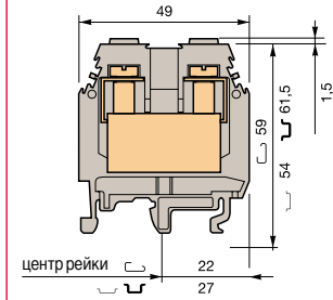
М 35/16
