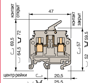
М 6/8.SNB
