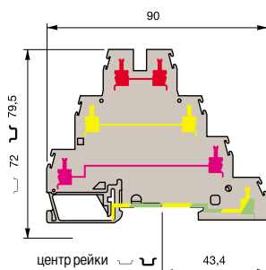
М 4/6.T3.P
