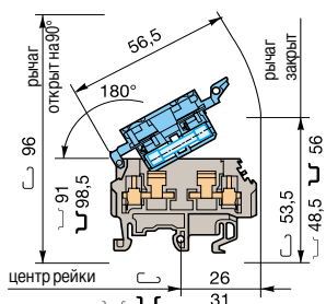
М 4/8.SN
