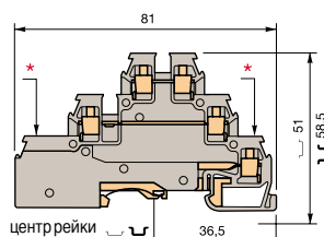
D 2,5/6.DPA1
