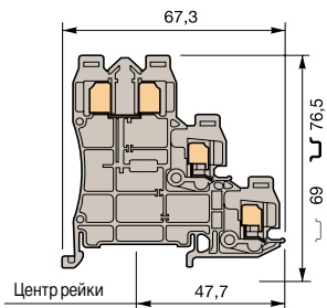
D 1/5.C3.ADO
