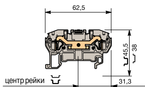
D 4/6.2L
