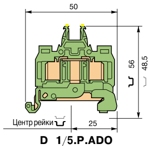
D 1/5.P.ADO
