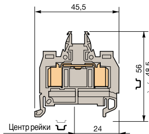
D 1,5/6... ADO
