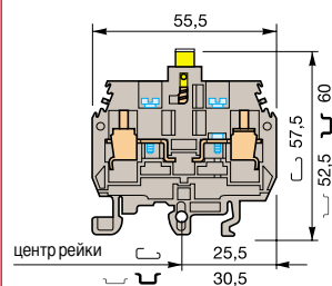
М 6/8.STP
