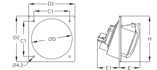
216-432RAU...
