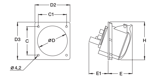
216-432RAM..
