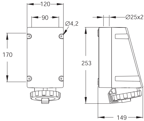
216-416RL..W 232-432RL..W
