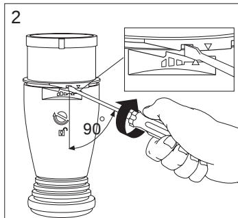
2. Поверните отвертку вправо до щелчка
