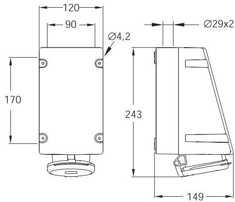
216-416RL.. 232-432RL..
