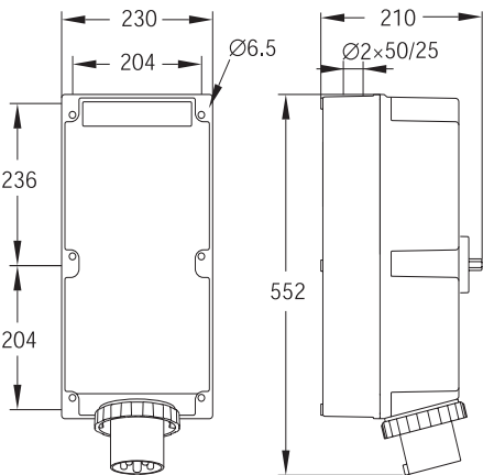
2125-4125BS...W
