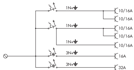
MP32/2
