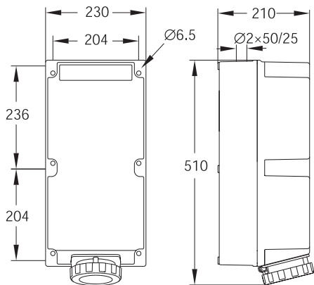
2125-4125RL..W
