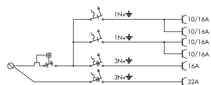
MPR32
