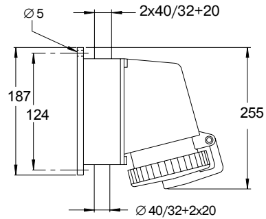
CUHV -63
