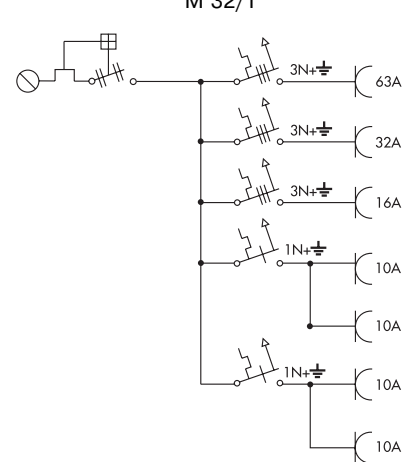
M 32/1
