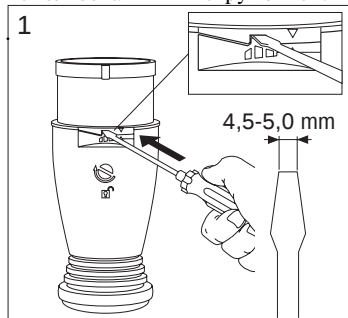
1. Вставьте отвертку в зазор, как показано выше.
