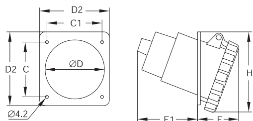
263-463RAU...W
