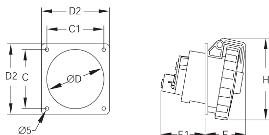
216-432RAU...W
