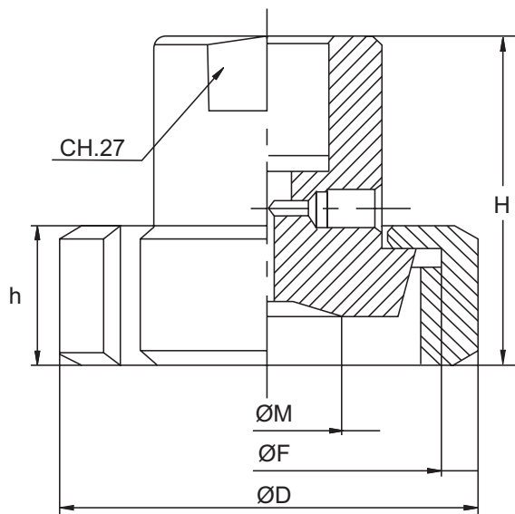
DIN 11851
