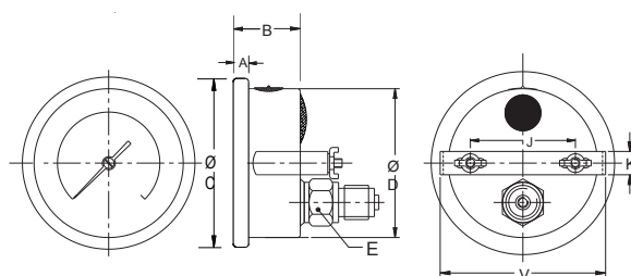
Исполнение ТЭС (осевое, эксцентричное, со скобой)
