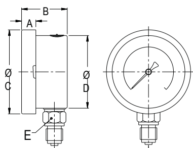
Исполнение Р (радиальное)
