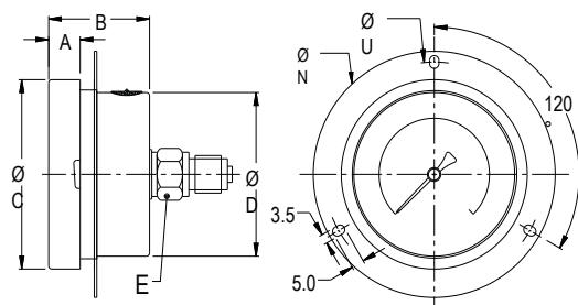
Исполнение ТГПФ (осевое, передний фланец)
