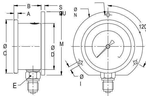
Исполнение РЗФ (радиальное, задний фланец)
