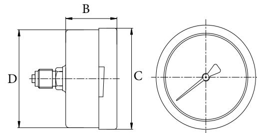
Исполнение Т (осевое, DIN корпус)
