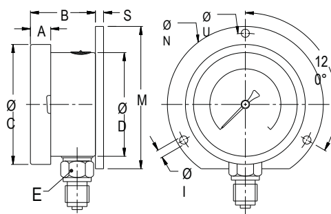
Исполнение РЗФ (радиальное, задний фланец)
