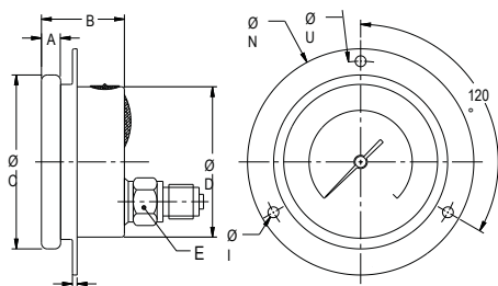
Исполнение ТЭПФ (осевое, эксцентричное, передний фланец)
