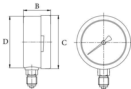
Исполнение Р (радиальное, DIN корпус)
