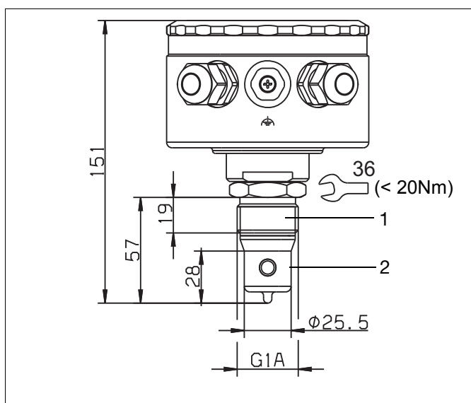
Исполнение с подключением к процессу 955 = прижимное соединение G 1" (⌚ < 20Nm) EL = 57 мм
