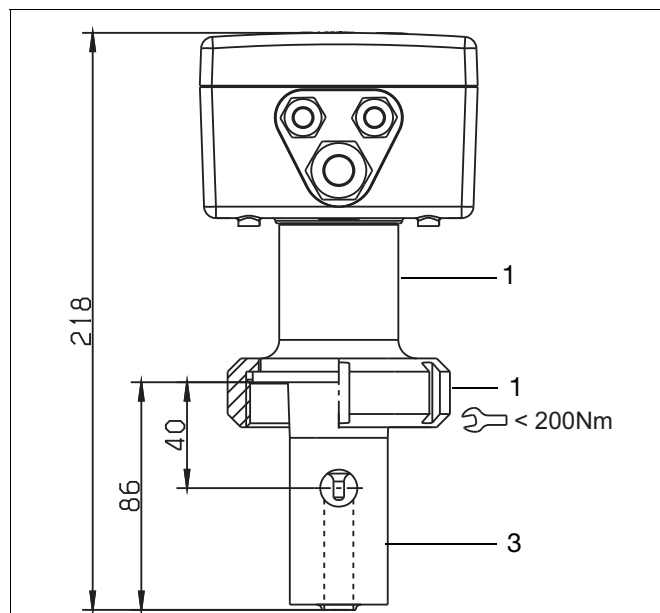
Исполнение с подключением к процессу 690 = SMS 2" (⌚ < 200Nm) и типовым дополнением 768
