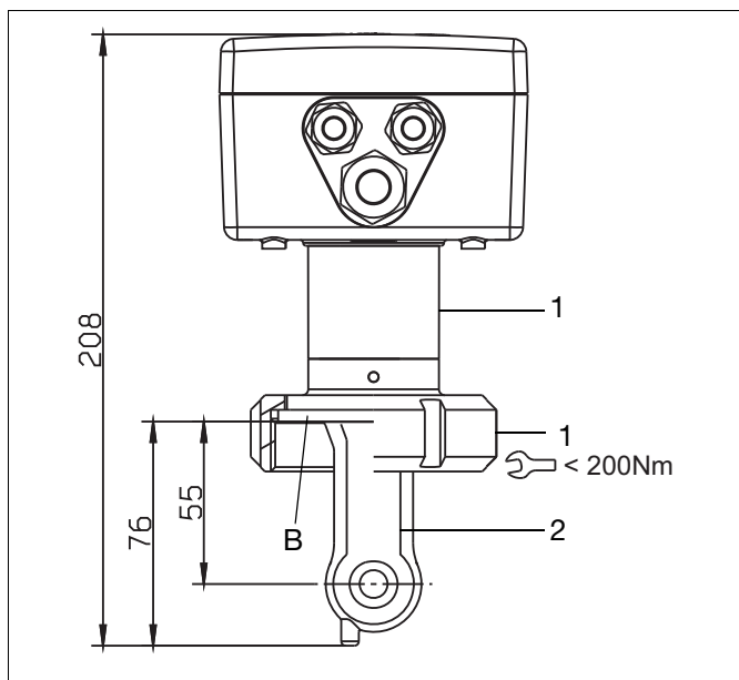
Исполнение с подключением к процессу 690 = SMS 2" (⌚ < 200Nm) и типовым дополнением 767 и 941
