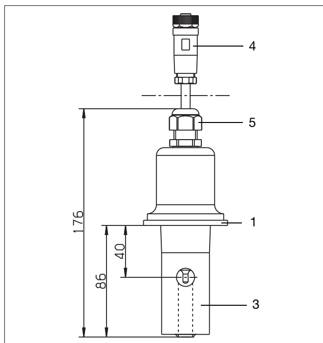
Раздельное исполнение с подключением к процессу 690 = SMS 2" ( \mathcal{C} < 200Nm) и типовым дополнением 768 (накидная гайка не входит в комплект поставки)
