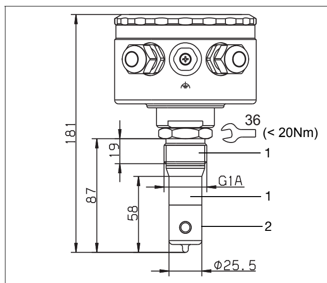
Исполнение с подключением к процессу 956 = прижимное соединение G 1" (⌚ < 20Nm) EL = 87 мм
