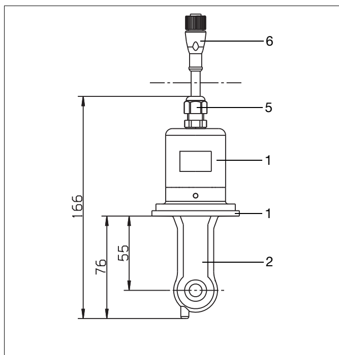
Раздельное исполнение с подключением к процессу 690 = SMS 2" ( \mathcal{C} < 200Nm) и типовым дополнением 767 и 941 (накидная гайка не входит в комплект поставки)
